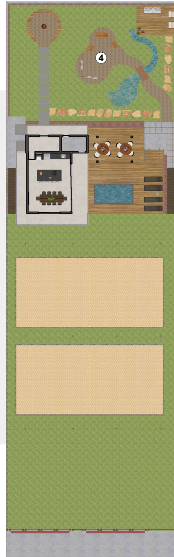
PLANTA BAIXA - PAVIMENTO SUPERIOR
