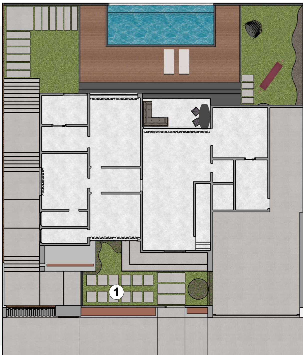
PLANTA BAIXA - PAV. TÉRREO
