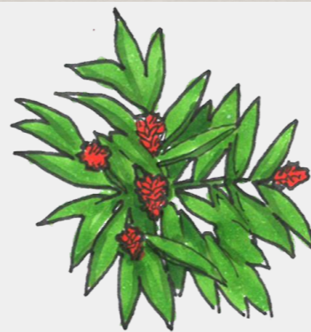
① Alpínia
